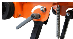
ÖSSZECUKHATÓ ÉS RÖGZÍTHETŐ LÁBAK
